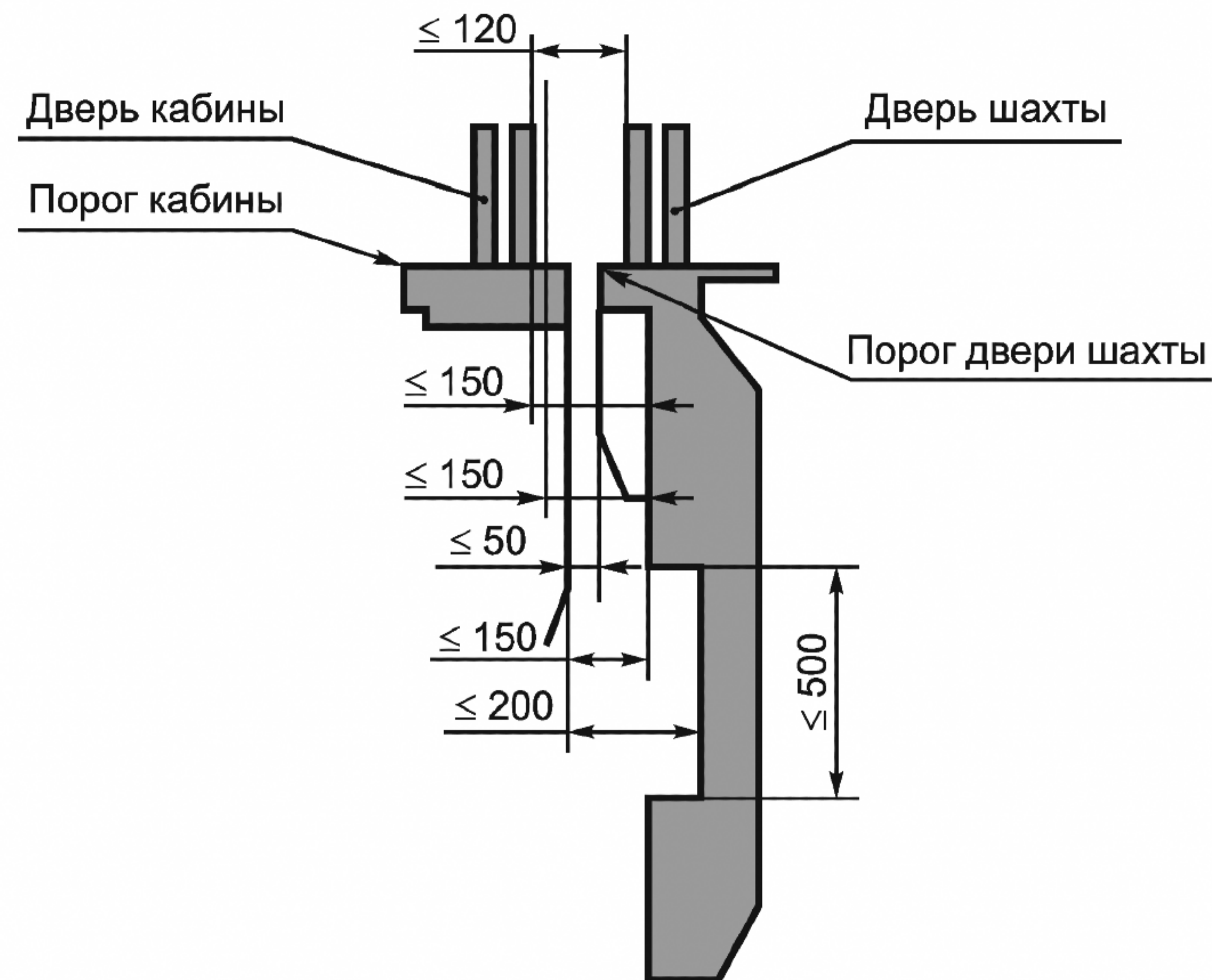
Рисунок 3 — Расстояние между элементами кабины и шахты
